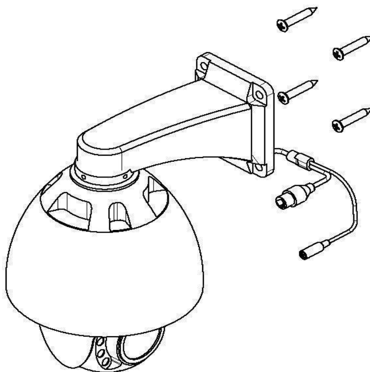
Рисунок 3.1 - Монтаж видеокамеры
