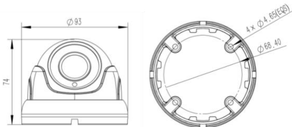
Рисунок 1.2 - Габаритные размеры видеокамеры
