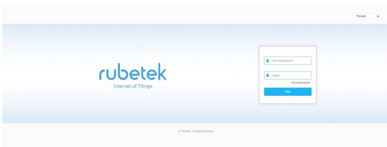
Рисунок 3.8 - Экран авторизации
