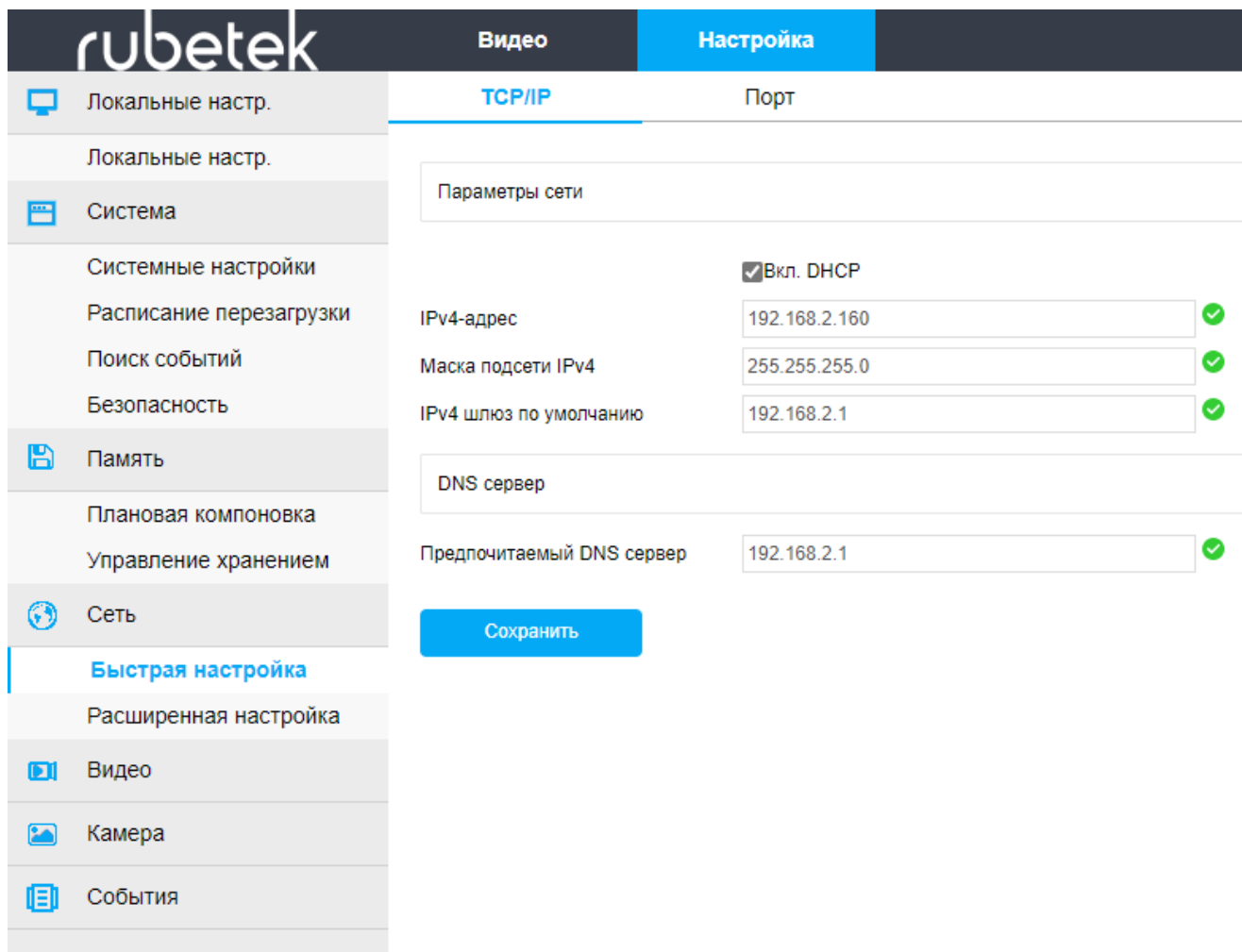
Рисунок 3.26 - Вкладка «TCP/IP»
