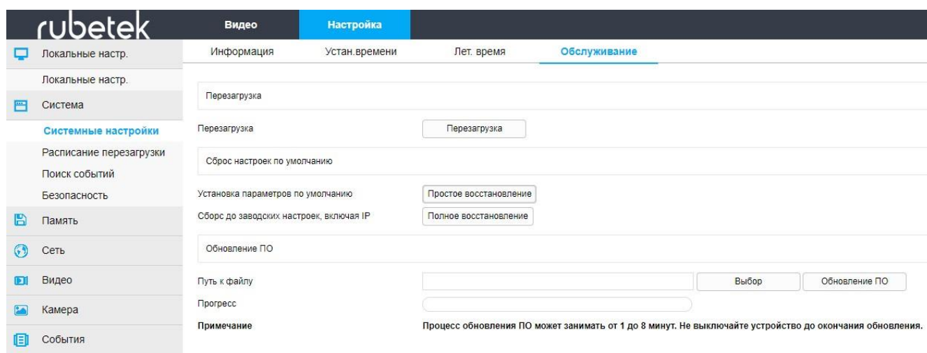
Рисунок 3.20 - Вкладка «Обслуживание»
