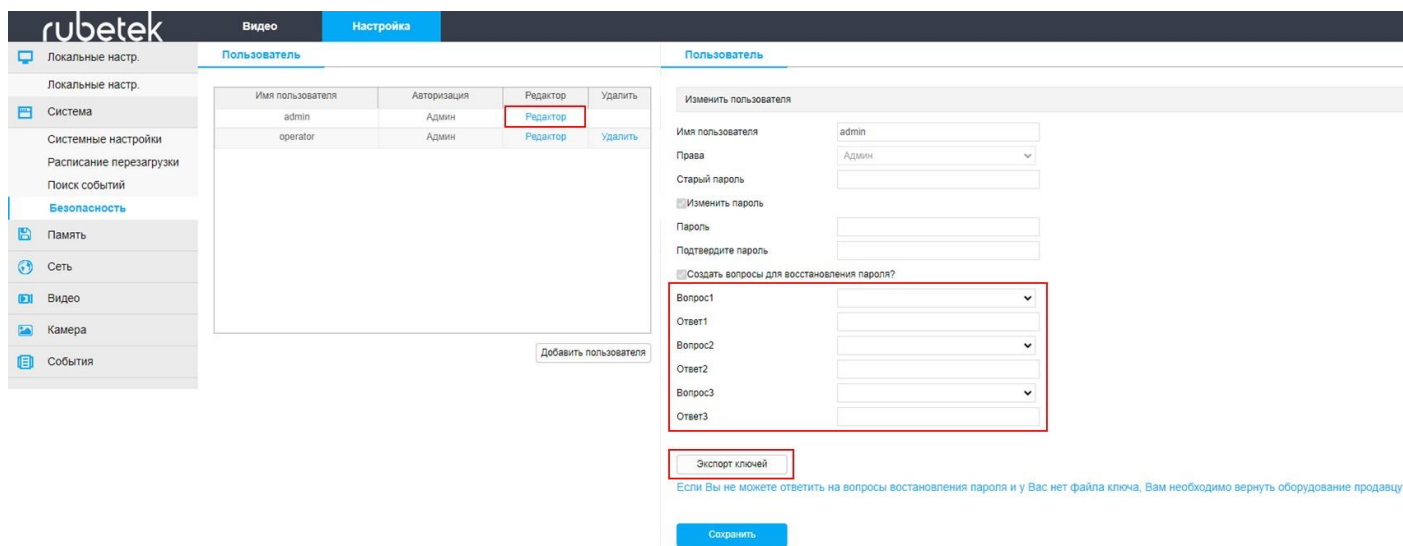
Рисунок 3.9 - Изменение пароля
