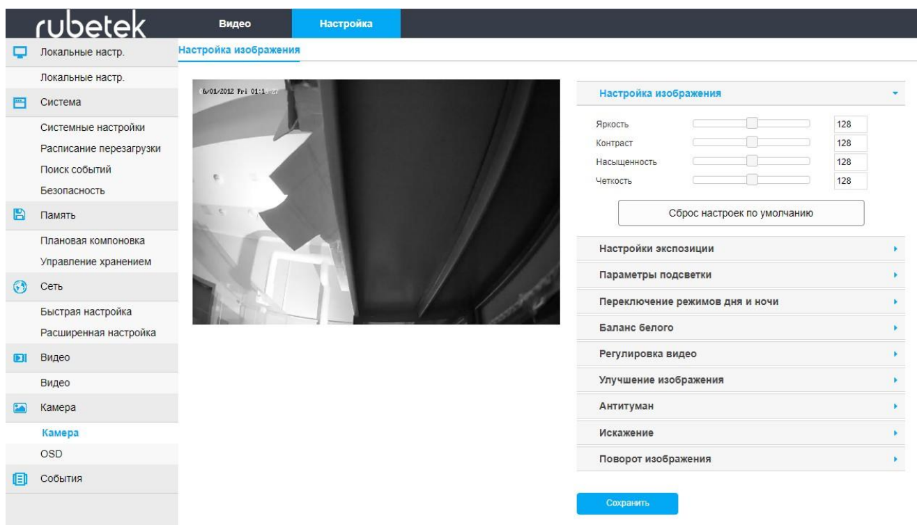
Рисунок 3.28 - Подраздел «Камера»
