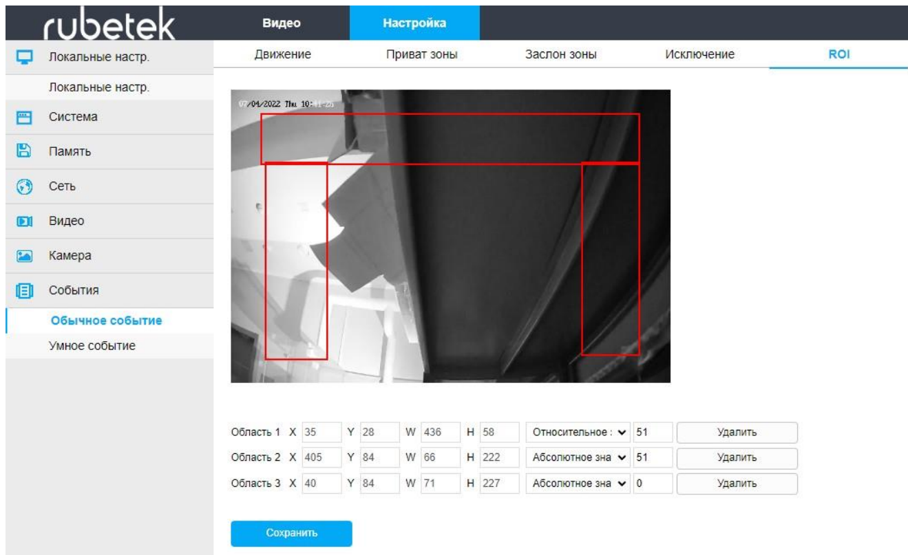
Рисунок 3.34 - Вкладка «ROI»
