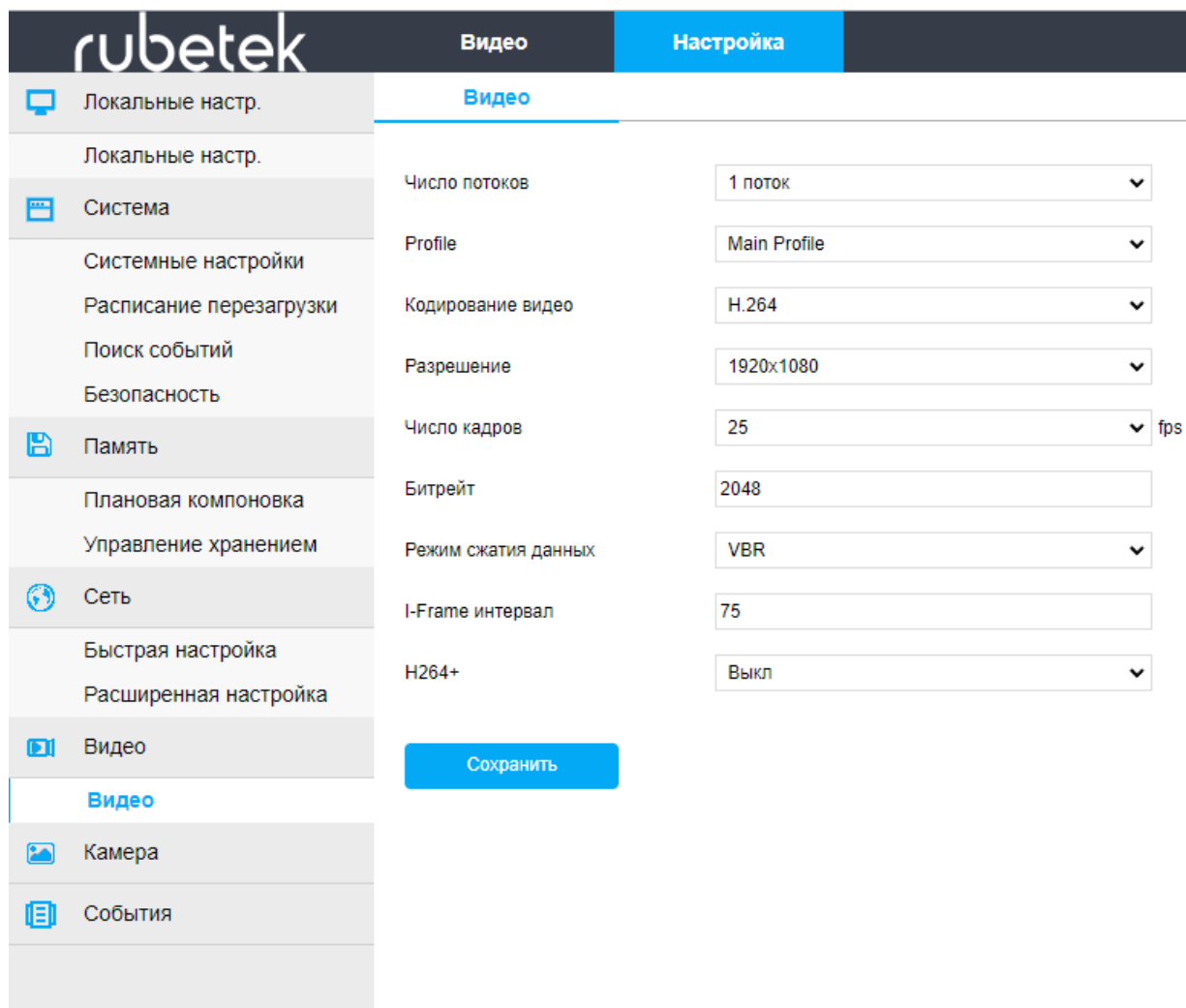
Рисунок 3.27 - Подраздел «Видео»
