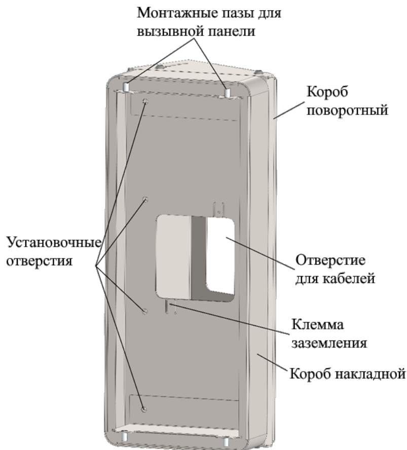
Рисунок 1 – Крепление поворотное
