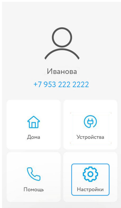
Блок «Настройки»
