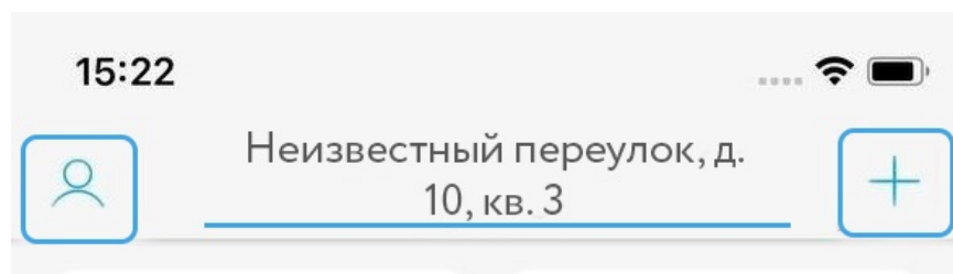
Панель настроек
