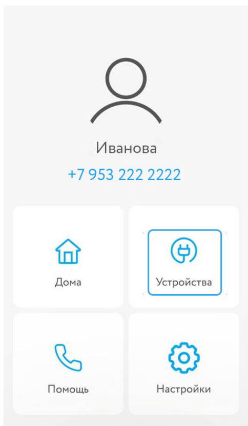
Блок "Устройства"
