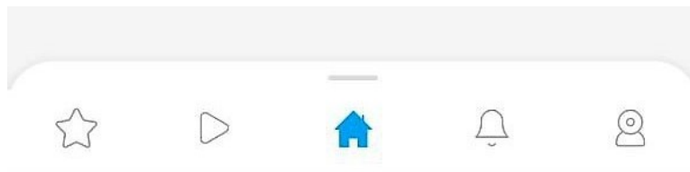
Разделы приложения
