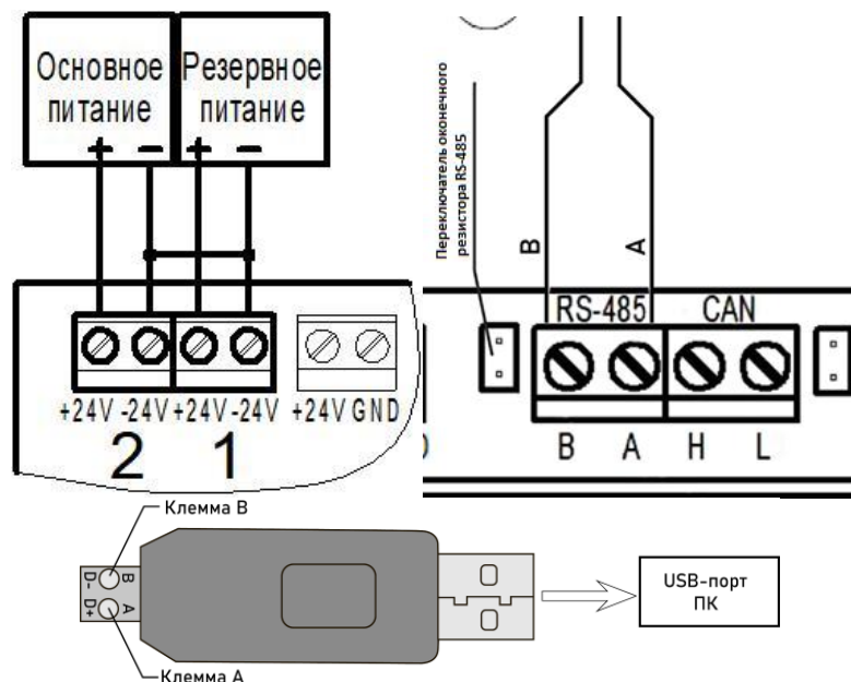
Рисунок 14 – Схема подключения адаптера USB-RS485
