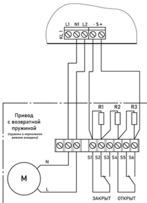
Рисунок 9 – Схема подключения привода с возвратной пружиной (пружина в нормальном режиме взведена, привод постоянно под напряжением)
