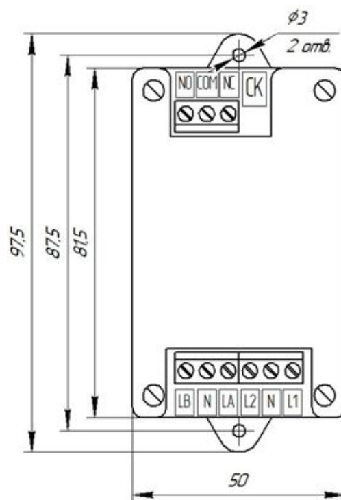
Рисунок 2 - Габаритные размеры МК-4
