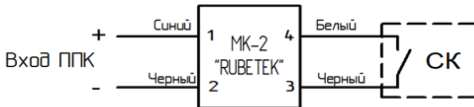
Рисунок 6 - Схема подключения СК
