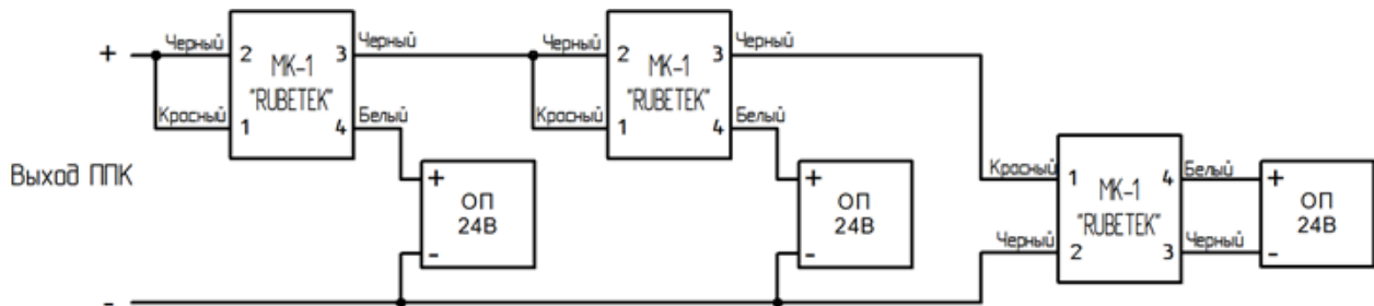
Рисунок 5 - Схема подключения нескольких ОП
