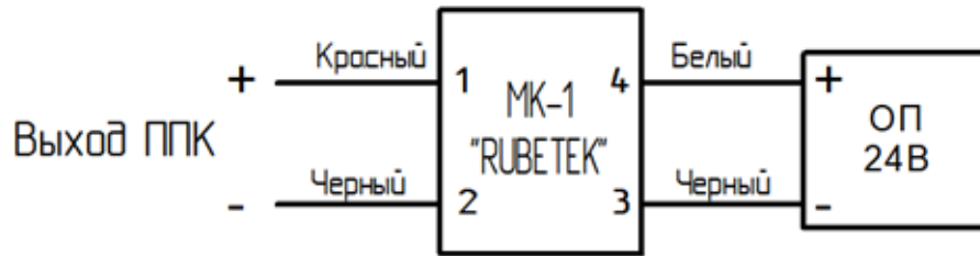
Рисунок 4 - Схема подключения одного ОП
