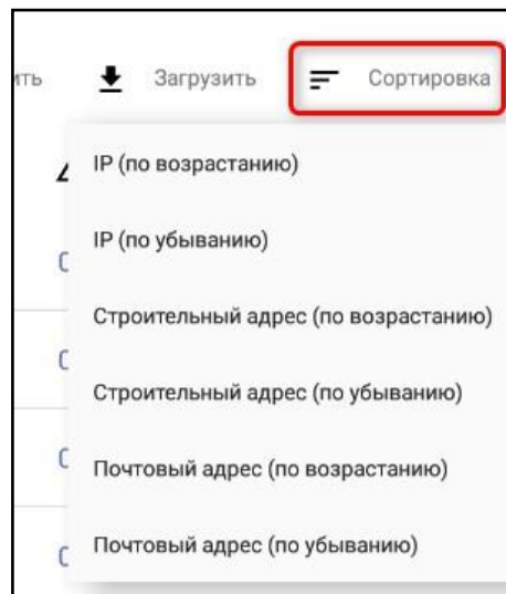
Рисунок 12 - Варианты сортировки
