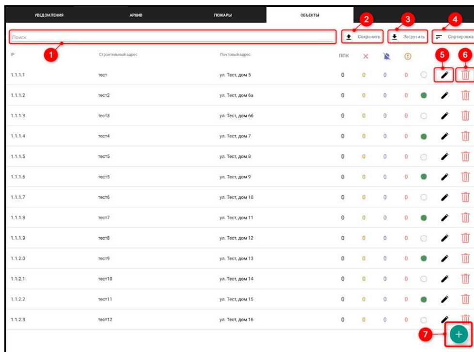
Рисунок 9 - Вкладка “Объекты”
