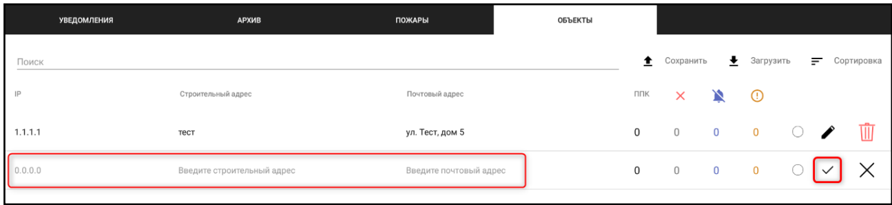
Рисунок 11 - Добавление объекта
