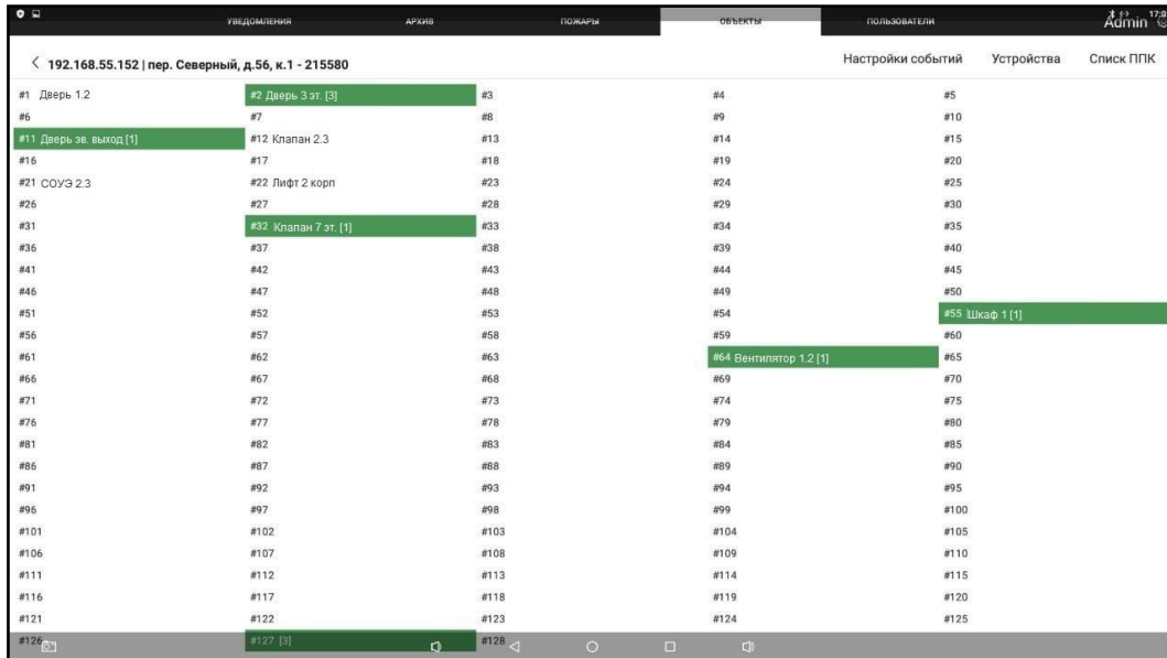
Рисунок 13 - Страница События
