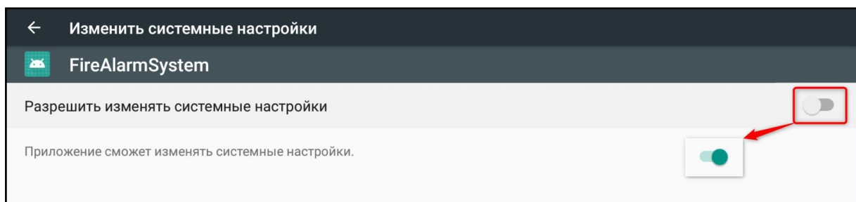
Рисунок 6 - Установка разрешения
